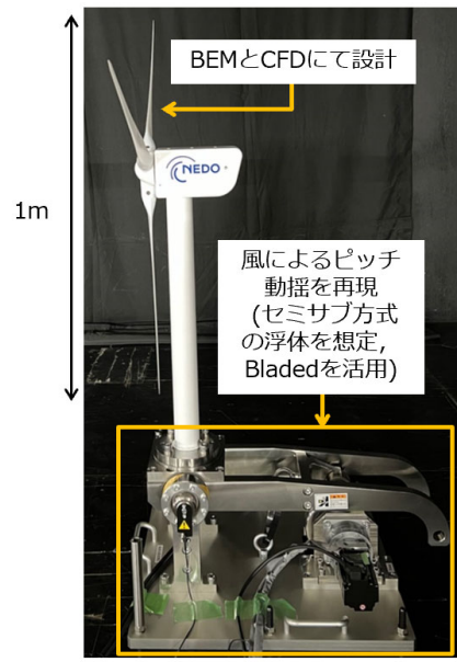
本PJで製作した15MW風車模型(1/240)と加振装置
